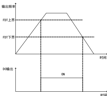
图 6-11 FDT 频率输出水平
