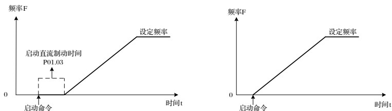
图 6-4 直接启动示意图
