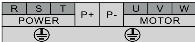
ES100 45KW-55KW 主回路端子示意图
