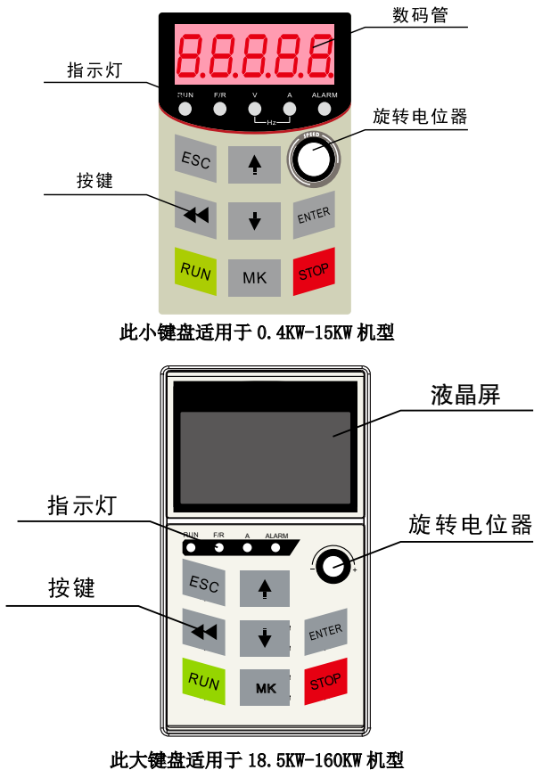
图 4-1 键盘介绍
