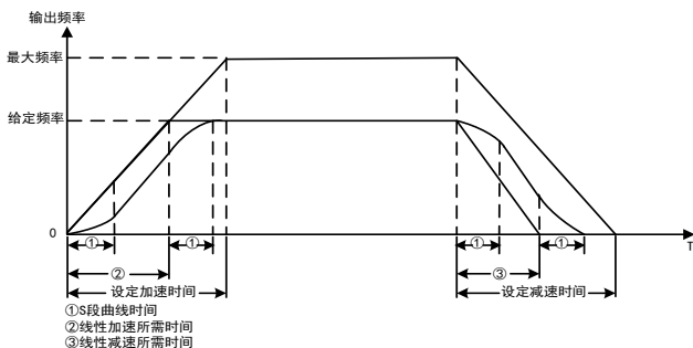
图 6-3 直线与 S 曲线加减速示意图
