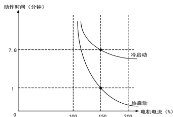
图 6-13 电机过载保护
