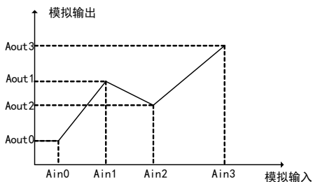
图 6-10 模拟输入偏置
