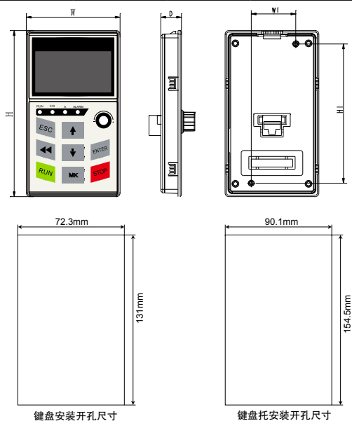
图 2-3 键盘尺寸图及键盘托尺寸图 (单位: mm)
