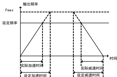
图 6-1 加减速时间
