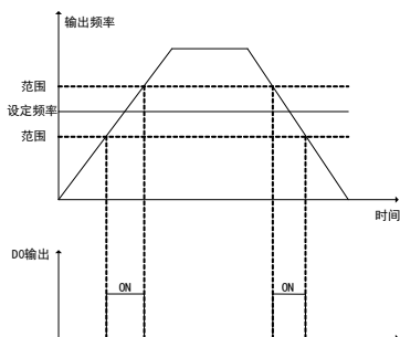
图 6-12 FAR 频率输出水平
