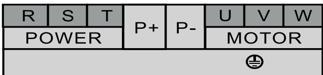
ES100 75KW-90KW 主回路端子示意图
