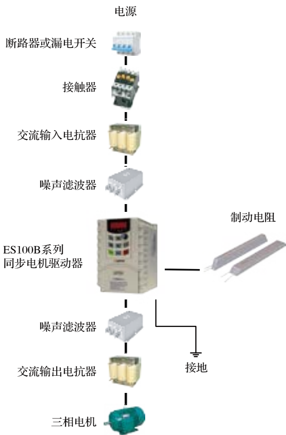
图 3-8 ES100B 系列变频器与外围设备的接线图
