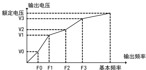
图 6-5 多点 V/F 曲线示意图
