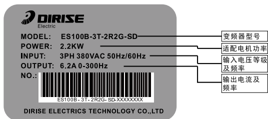
图 2-2 变频器铭牌
