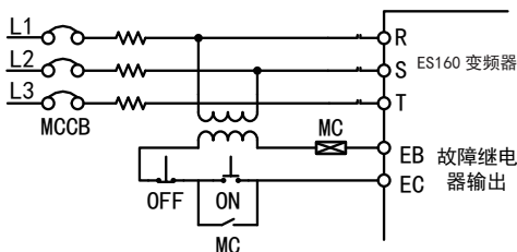
图 3-11 主回路断路器配线图
