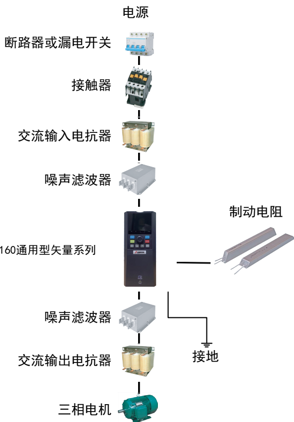
图 3-8 ES160 系列变频器与外围设备的接线图
