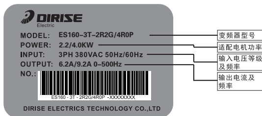
图 2-2 变频器铭牌
