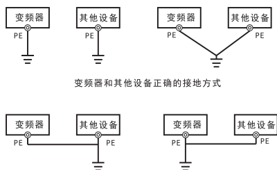
图 8-2 变频器和设备不推荐的接地方式
