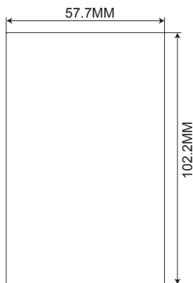
键盘托安装开孔尺寸
