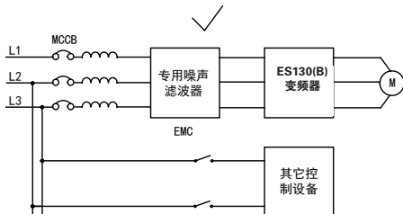
图 3-12 噪声滤波器正确安装配线
