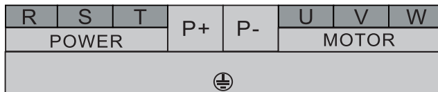
ES130(B) 110KW 主回路端子示意图
