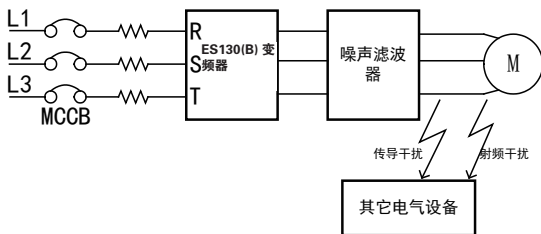
图 3-14 输出侧噪声滤波器安装配线
