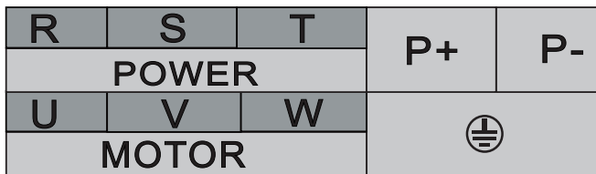
ES130(B) 132KW-160KW 主回路端子示意图
