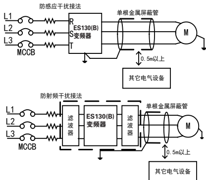
图 3-15 抗干扰安装配线
