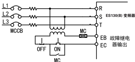
图 3-11 主回路断路器配线图
