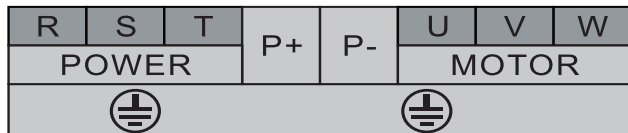
ES130(B) 45KW-55KW 主回路端子示意图
