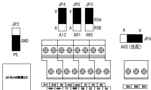
图 3-17 控制回路端子
